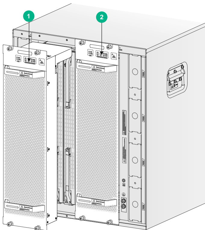
图3-3 风扇框上的网板指示灯与网板槽位对应关系（以 S12600-08-G 为例）
